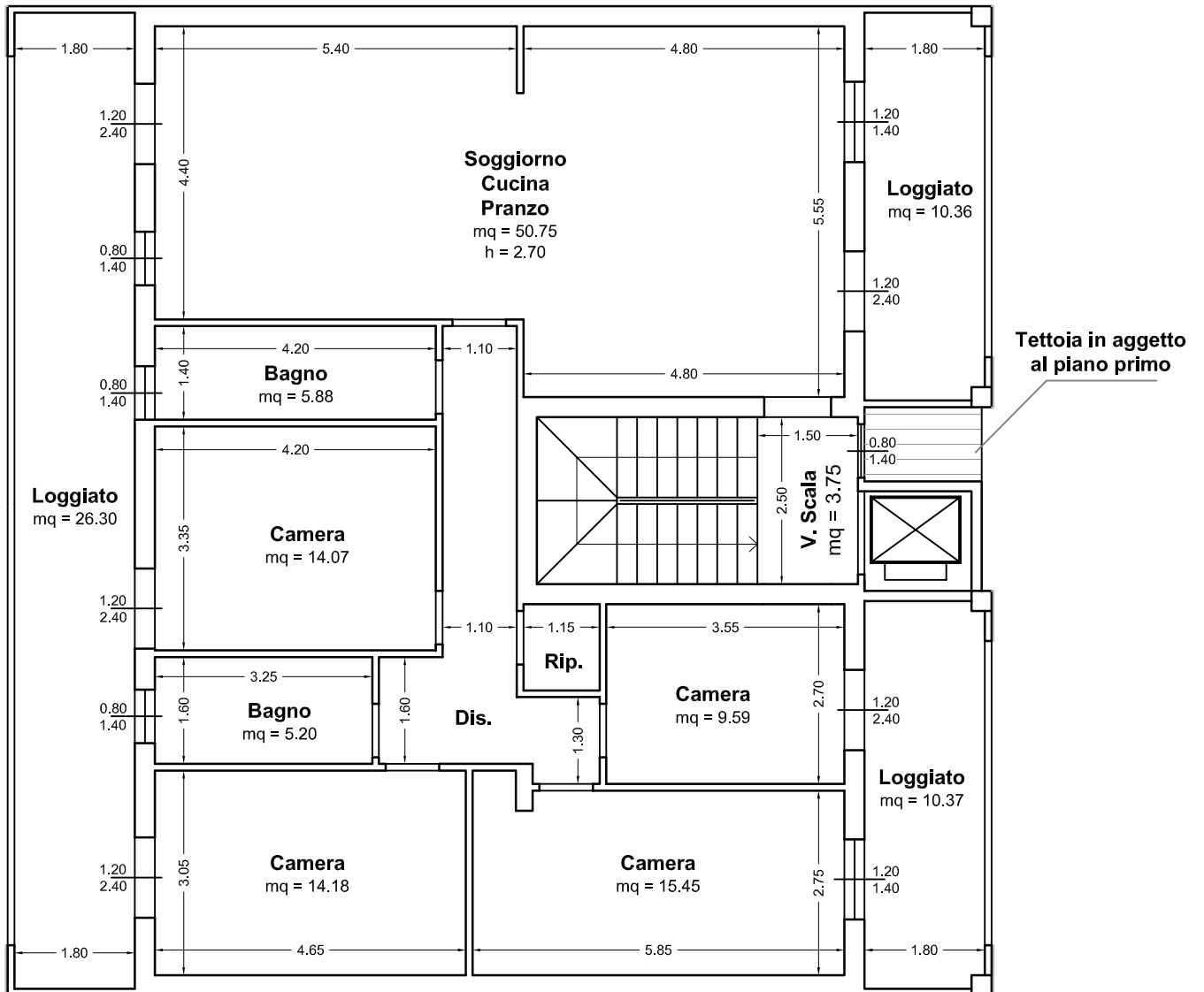
PIANTA PIANO TIPO SOLUZIONE UNICO APPARTAMENTO SCALA 1:100 - STATO PROGETTO
